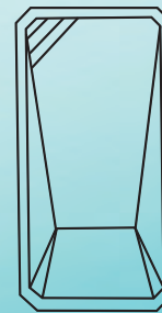
DELOS L 8,50 m x l 4,00 m Petit bain 1,20 m Grand bain 2 m
