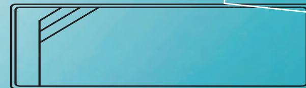
COULOIR DE NAGE L 11,00 m x l 3,00 m Prof. 1,50 m Fond plat
